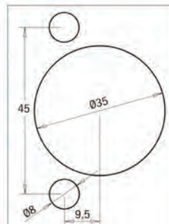
2 CMT333-4595 per cerniera Blum 45/9,5 para bisagra Blum 45/9,5
